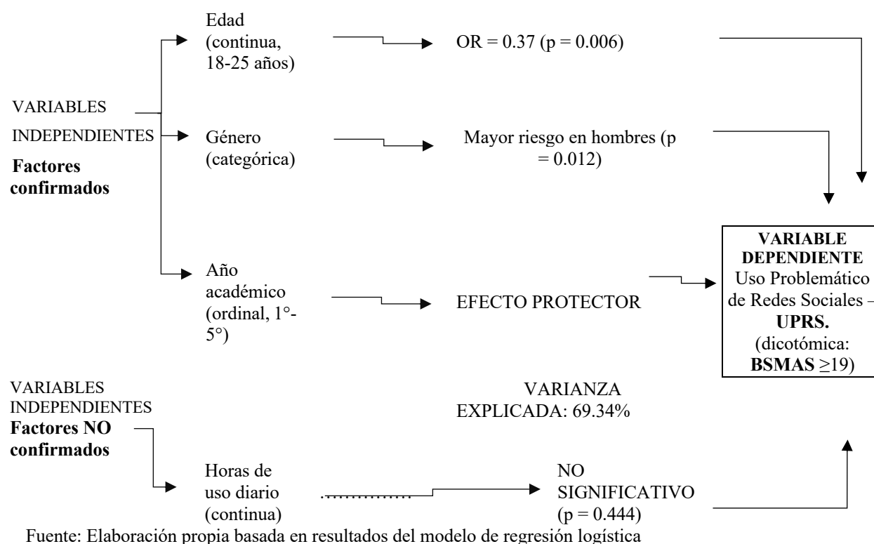
Figura 4. Modelo predictivo ex-post - resultados del análisis de regresión logística
