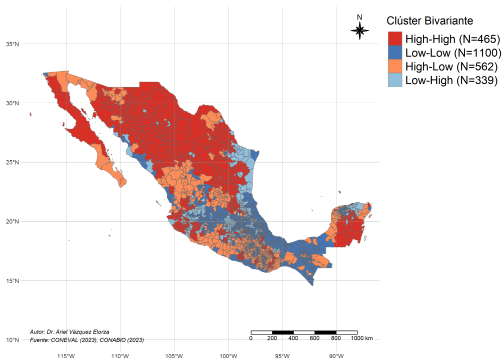
Figura 7 Clúster Bivariante del Índice Global de Moran
